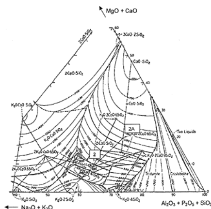
2 Popel z pšeničné slámy bez aditiva 2A Popel z pšeničné slámy s aditivem
