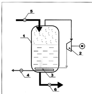
1 - tlaková nádoba 2 - kompresor 3 - kondenzátor destilátu 4 - čerpadlo 5 - čerpadlo 6 - čerpadlo
