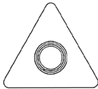
6.2
