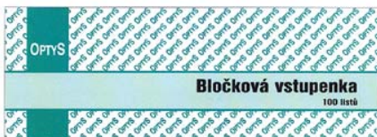
4.1
