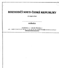
4.1
