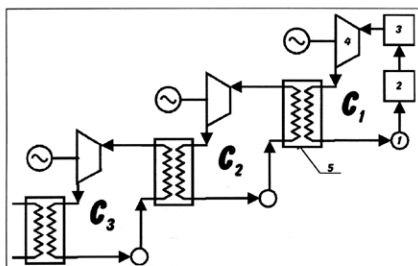
1-čerpadlo, 2-parní generátor, 3-parní přehříváč, 4-parní turbína, 5-výměník
